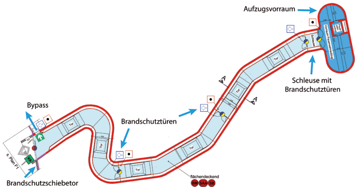
Bild 19: Grundriss des Tunnels
